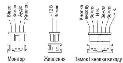
Розташування проводів в роз'ємах
