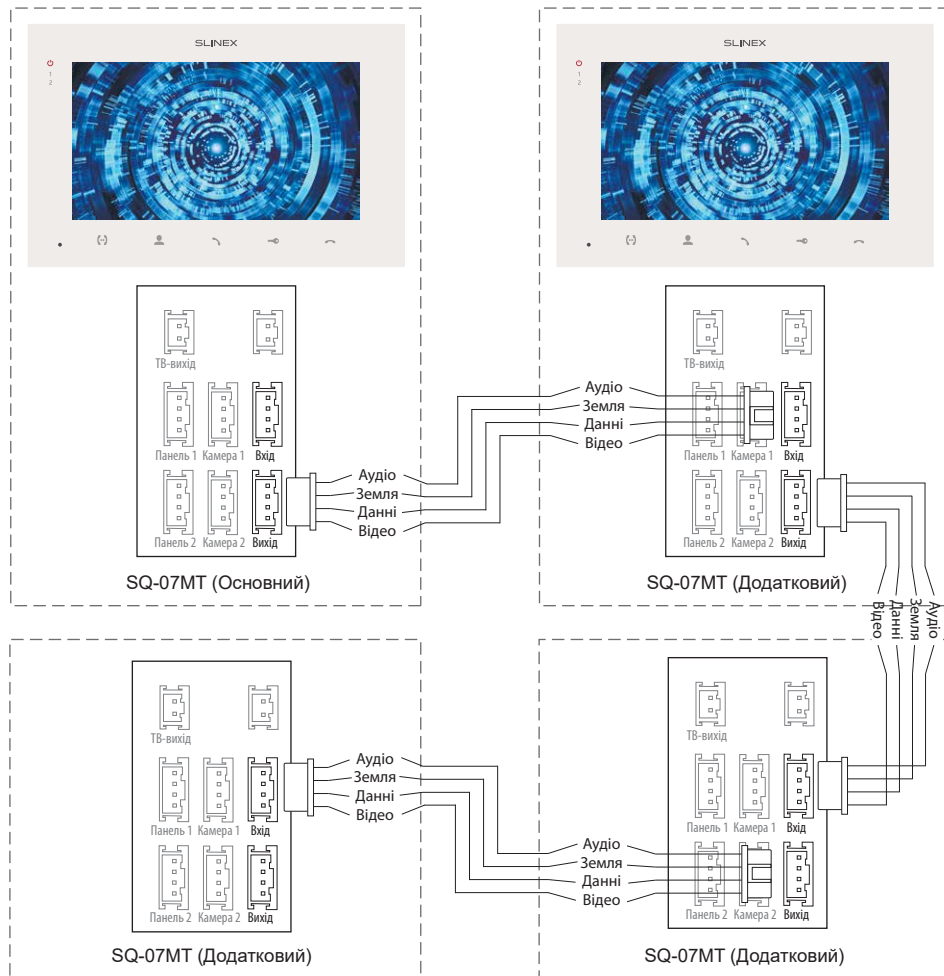
Схема 2. Підключення системи домофонів SQ-07MT.
